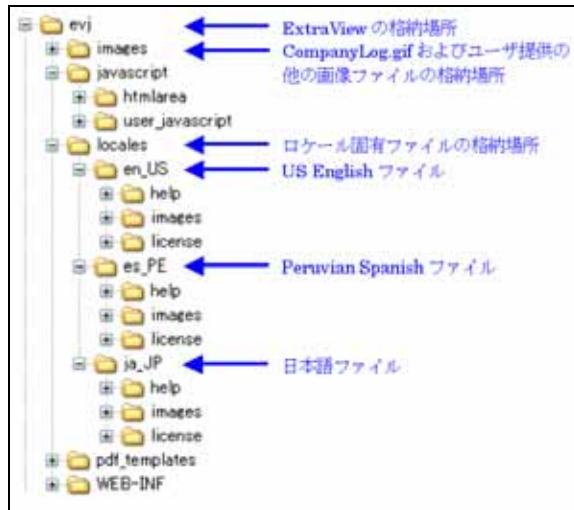
ディレクトリ構造
