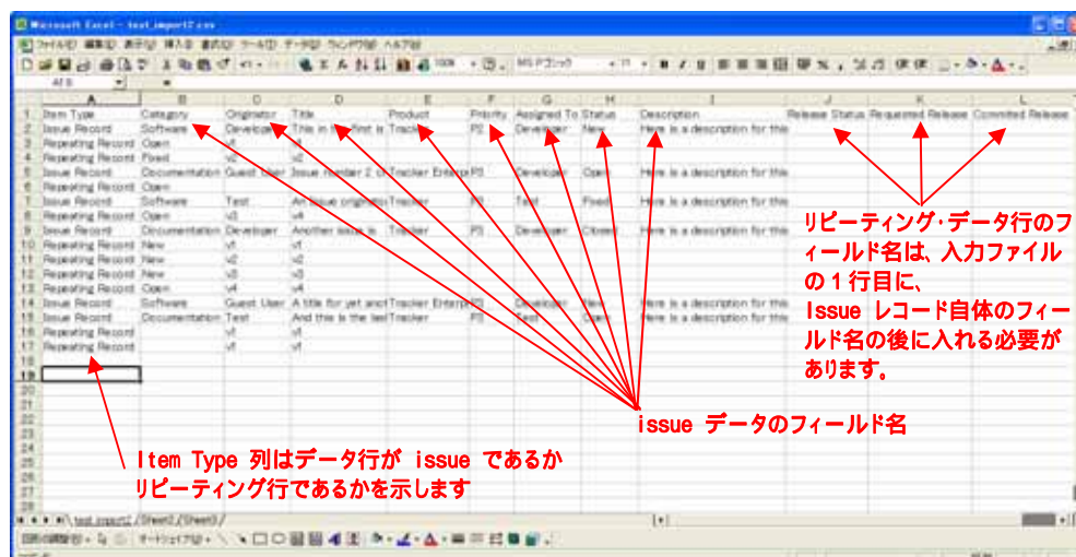
リピーティング行データのあるインポート・ファイル
