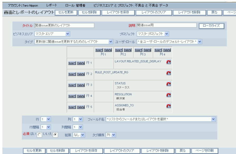
関連 issue の更新のレイアウト
