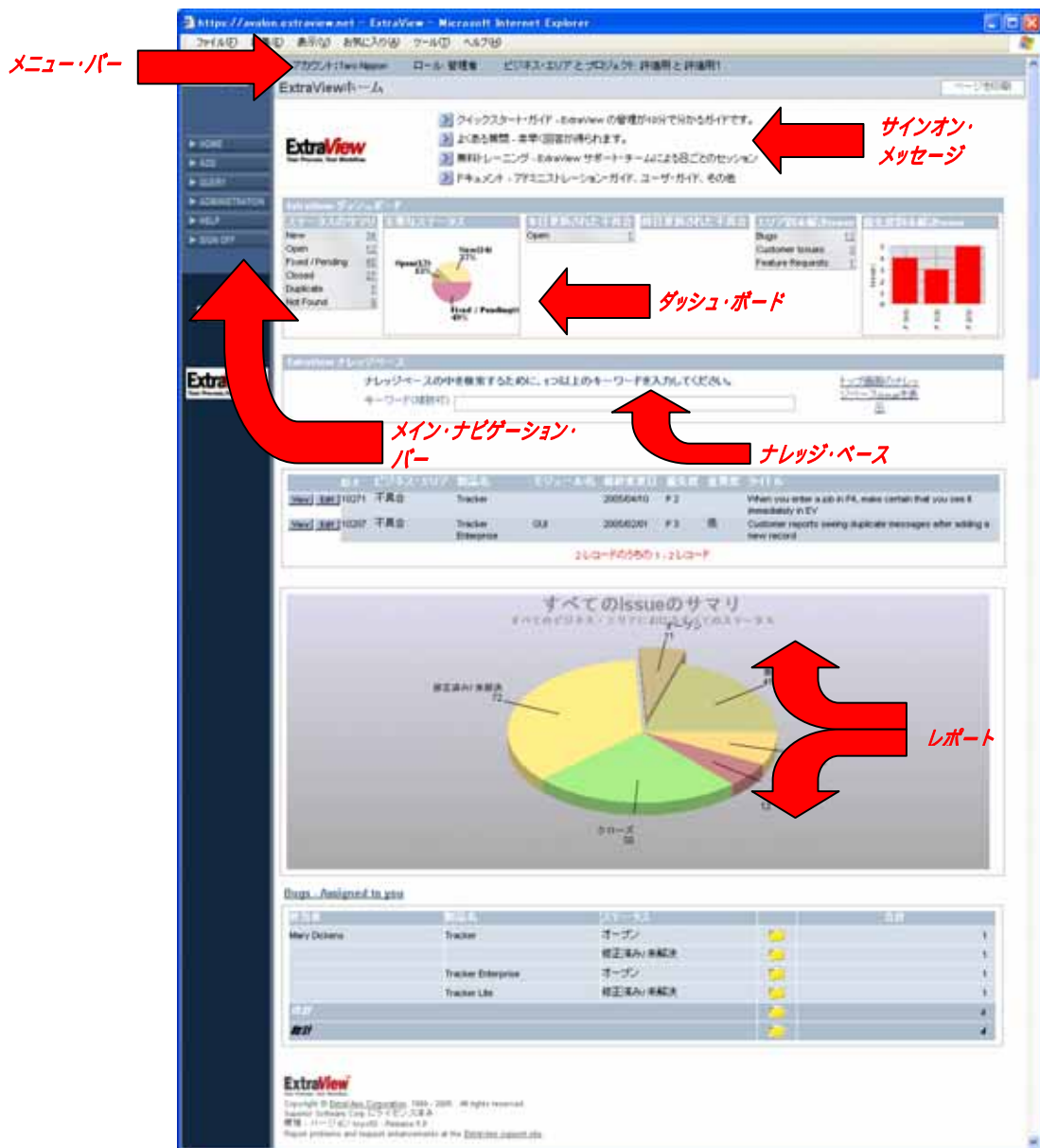
ホーム・ページ画面
