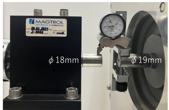
軸合わせ治具取り付けイメージ
