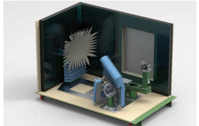
mini Mobile CATR ソリューション
