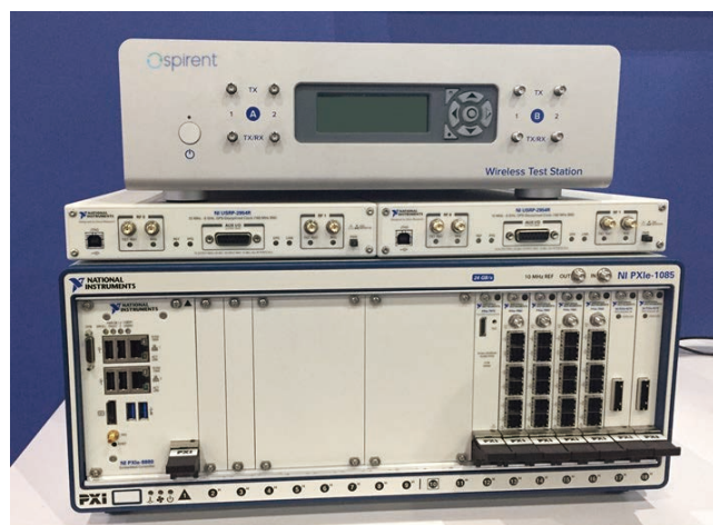
【5G NSAシミュレーションシステム】
