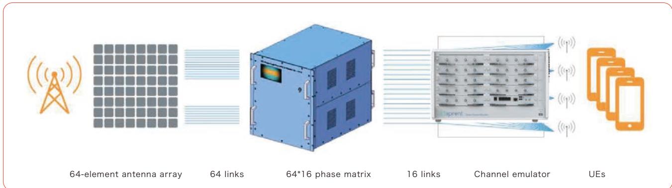
組み合わせ試験系の例(Spirent Vertex)との組み合わせ
