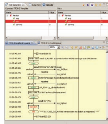
SUPL 2.0 シーケンス解析ツール
